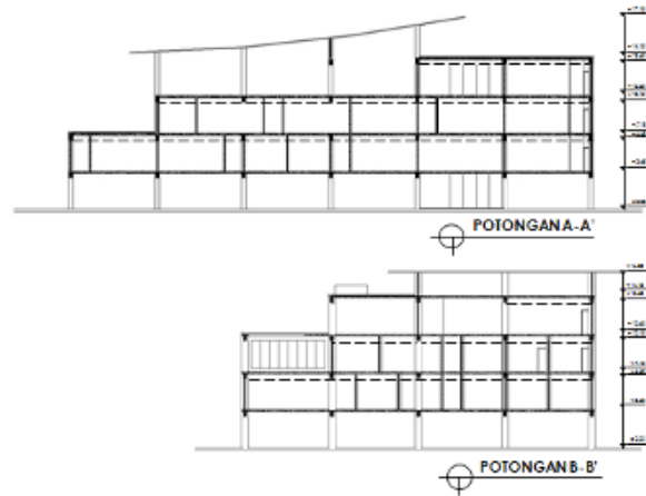
Gambar 10. Potongan
