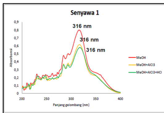
Gambar 3. Spektrum UV senyawa 1 pada MeOH, MeOH+AlCl 3 , dan MeOH+AlCl 3 +HCl.
