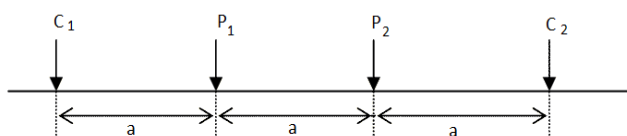
Gambar. 2. Penempatan elektroda konfigurasi Wenner.
