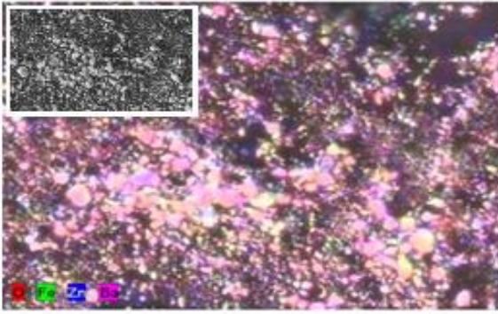
Gambar 3. Hasil Pengujian SEM EDX pada Material BAM
