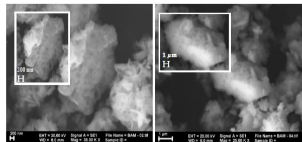
Gambar. 2. Hasil Pengamatan SEM pada Material BAM
