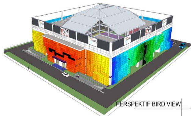
Gambar 7. Perspektif
