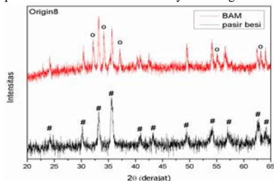
Gambar 3.2 Pola Difraksi Barium M-Heksaferit
