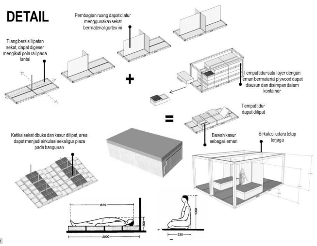
Gambar 4.10 Detail tempat tidur dan sekat ruang pada hostel
