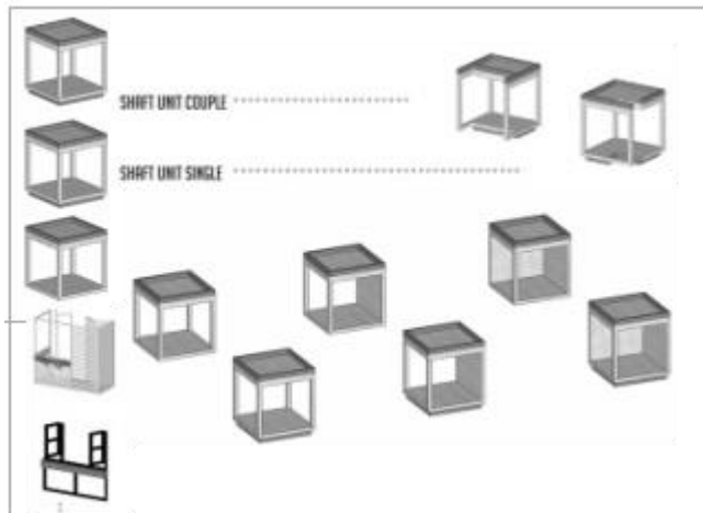
Gambar 2. Terdapat 3 jenis modul utama, 2 jenis modul dengan fungsi sebagai shaft dan 2 jenis modul sebagai elemen bukaan dengan konsep interlocking dan sistem struktur box.
