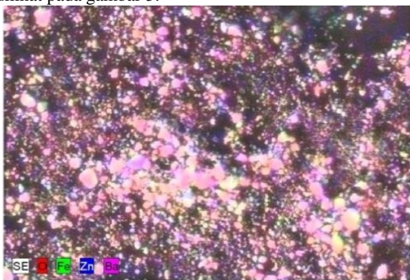
Gambar 5. Penyebaran komposisi penyusun BaM menggunakan SEM-EDX
