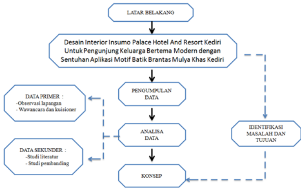
Gambar 2. Proses Desain
