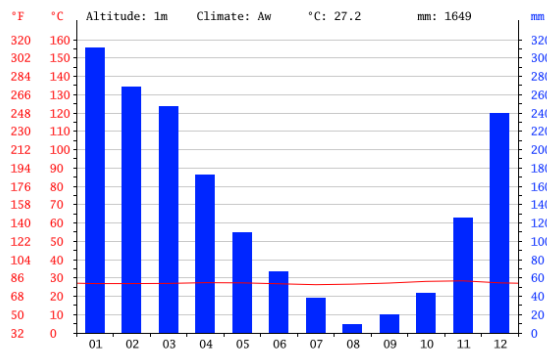
Gambar 1. Grafik Iklim
