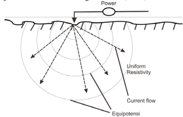
Gambar.3. Titik sumber arus pada media homogen [3]
