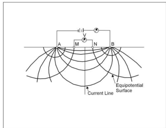
Gambar.4.Garis ekuipotensial arus antara elektroda pada media homogen [2]
