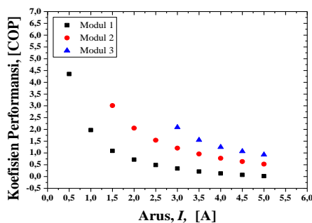
Gambar 4. Koefisien Performansi Modul Termoelektrik Cooler
