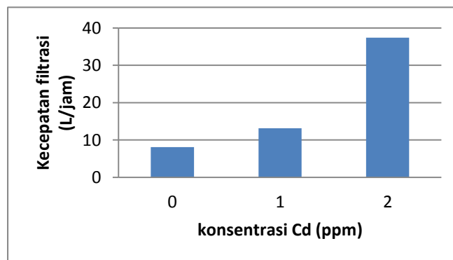
Gambar 2. Grafik rata-rata kecepatan filtrasi Perna viridis terhadap mikro alga Chaetoceros sp. pada media tercemar logam Cd.
