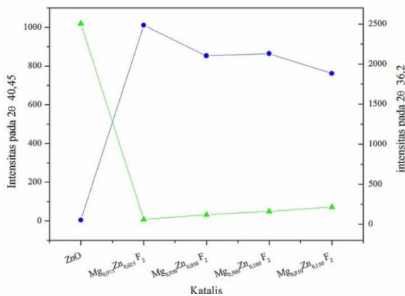
Gambar. 5. Intensitas Katalis Mg_{1-x}Zn_xF_2 terhadap 2\theta 40,45 yang merupakan puncak tertinggi MgF_2 dan terhadap 2\theta 36,2 yang merupakan puncak tertinggi ZnO.
