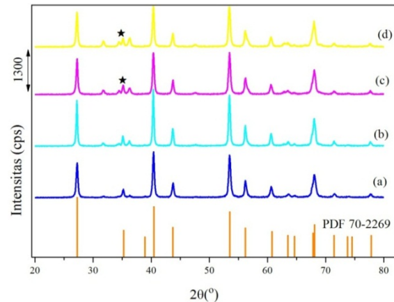
Gambar. 3. Difraktogram Katalis Mg 1-x Zn x F 2 (a) x = 0,025 (b) x = 0,05 (c) x = 0,10 (d) x = 0,15
