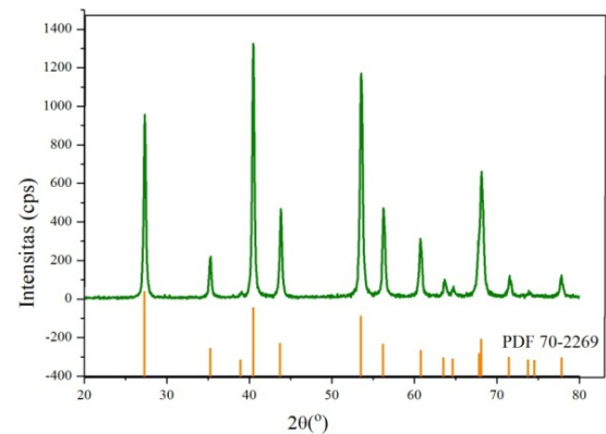
Gambar. 4. Difraktogram Katalis MgF 2
