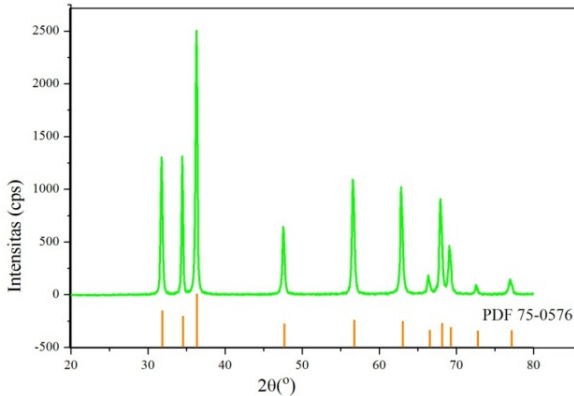
Gambar. 1. Difraktogram Katalis ZnO
