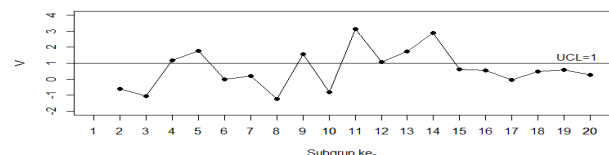
Gambar 8. Diagram kendali dengan the 3-of-3 test fase II.
