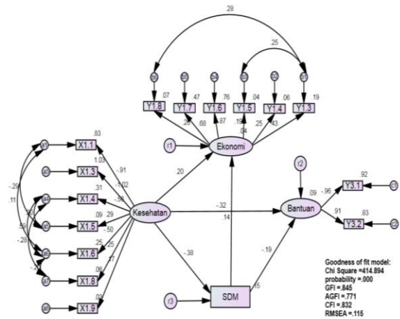
Gambar. 3. Model Struktural Setelah Modifikasi
