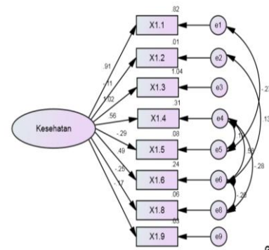
Gambar. 1. CFA Variabel Kesehatan Modifikasi
