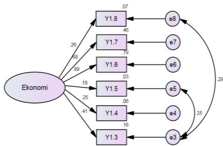
Gambar. 2. CFA Variabel Ekonomi Modifikasi
