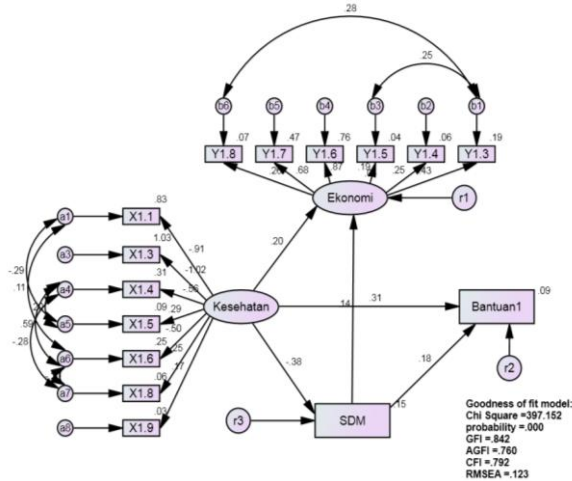
Gambar. 4. Model Struktural Bantuan 1 Modifikasi dan Signifikan
