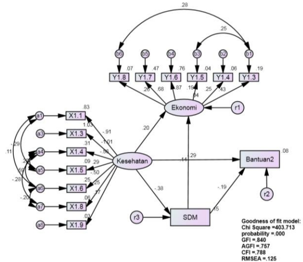
Gambar. 5. Model Struktural Bantuan 2 Setelah Modifikasi dan Signifikan
