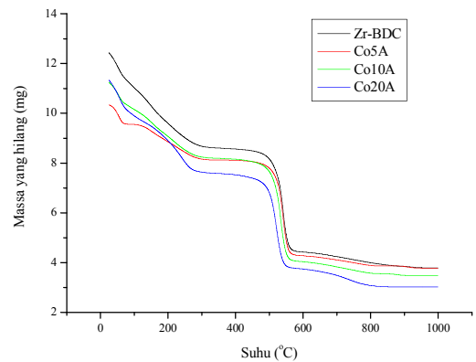
Gambar 4 Kurva TGA
