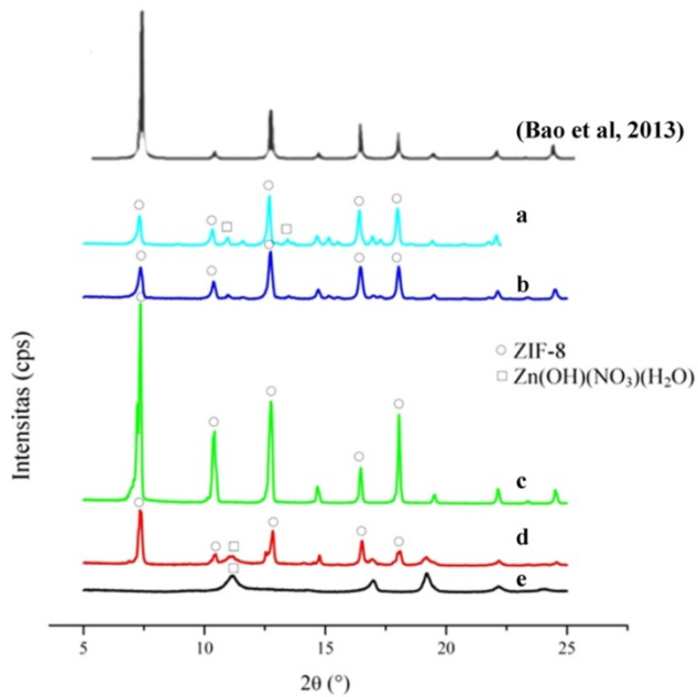
Gambar 1 Pola XRD sampel yang disintesis dengan variasi perbandingan molar \text{Zn}^{2+} -MeIM: (a) ZIF-8(1:3); (b) ZIF-8(1:2,5); (c) ZIF-8(1:2); (d) ZIF-8(1:1,5) dan (e) ZIF-8(1:1)
