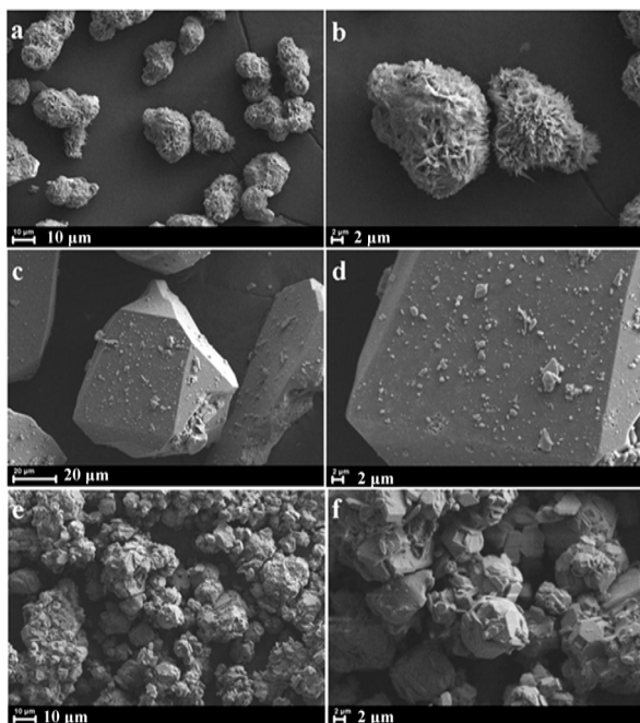
Gambar 3 Morfologi permukaan produk yang disintesis dengan variasi perbandingan molar Zn^{2+} -MeIM: (a,b) ZIF-8(1:1); (c,d) ZIF-8(1:2); dan (e,f) ZIF-8(1:3)
