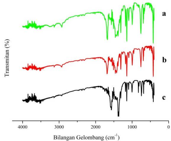
Gambar 2 Spektra FTIR sampel yang disintesis dengan variasi perbandingan molar \text{Zn}^{2+} -MeIM: (a) ZIF-8(1:3); (b) ZIF-8(1:2); dan (c) ZIF-8(1:1)
