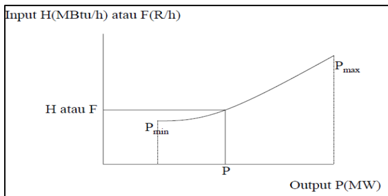
Gambar 1. Karakteristik input – output pembangkit termal
