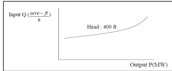
Gambar 2. Kurva input – output pembangkit hidro
