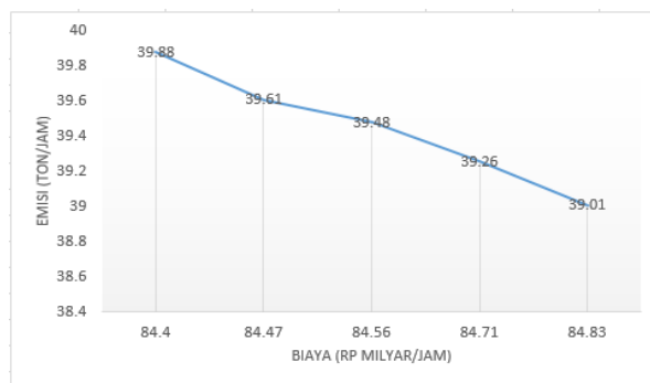
Gambar 7. Grafik Hubungan Biaya Pembangkitan dan Emisi Pukul 19.00
