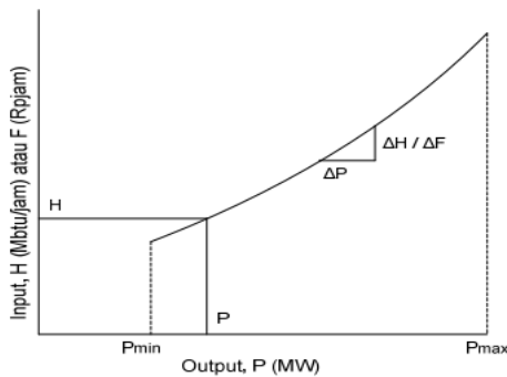
Gambar 1. Kurva Karakteristik Input-Output Unit Termal
