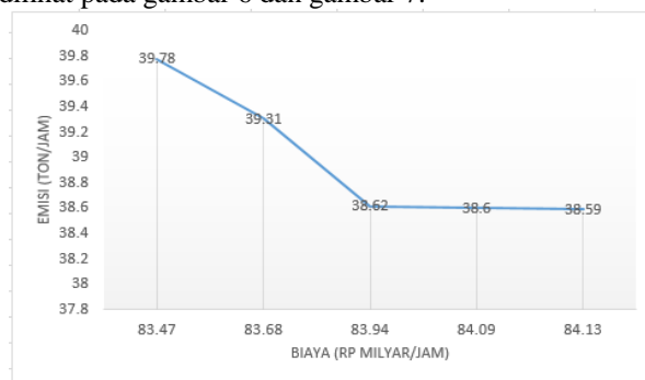
Gambar 6. Grafik Hubungan Biaya Pembangkitan dan Emisi Pukul 13.00
