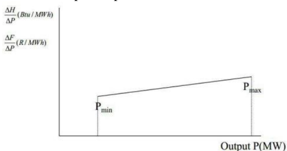
Gambar 2. Kurva Karakteristik Kenaikan Biaya/Panas Unit Termal
