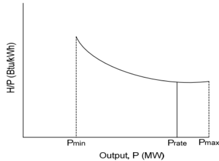
Gambar 3. Kurva Karakteristik Efisiensi Terhadap Output
