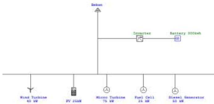
Gambar 2. Sistem kelistrikan micro grid
