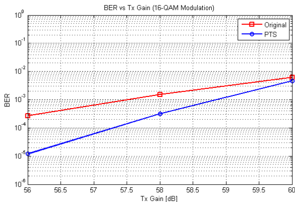
Gambar 8. Perbandingan Kurva BER Modulasi 16-QAM
