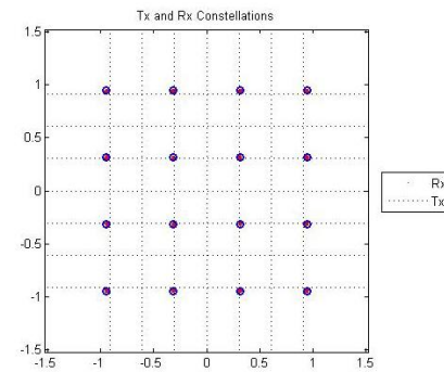
Gambar 11. Konstelasi Tanpa Distorsi Nonlinear
