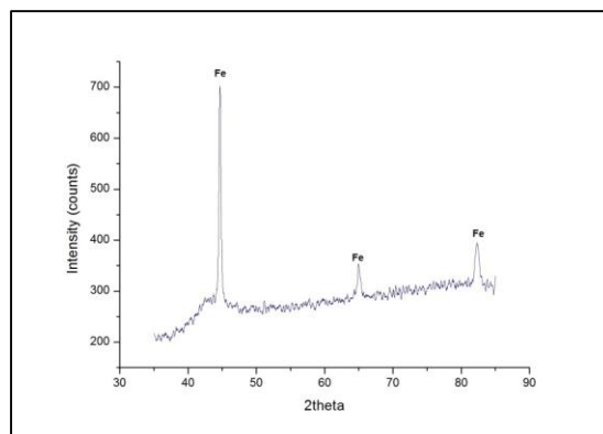
Gambar 3. Grafik Hasil XRD Baja AISI 1006
