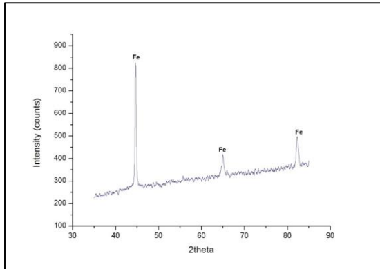
Gambar 4. Grafik Hasil XRD Copperized -AISI 1006
