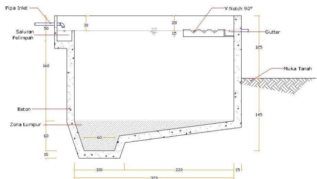
Gambar 4. Potongan Bak Prasedimentasi Tanpa Skala
