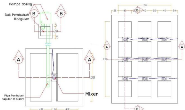
Gambar 5. Denah Unit Koagulasi – Flokulasi Tanpa Skala
