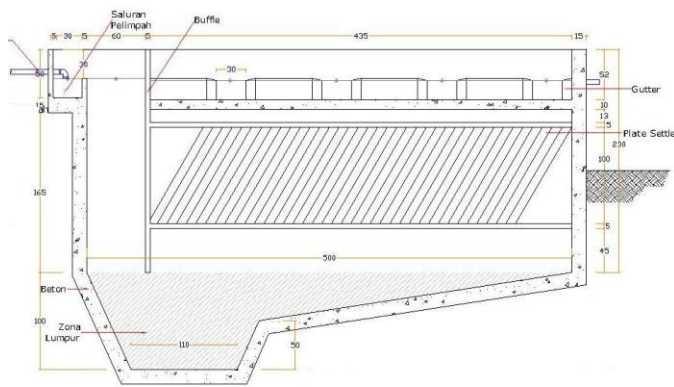
Gambar 6. Potongan Unit Sedimentasi Tanpa Skala
