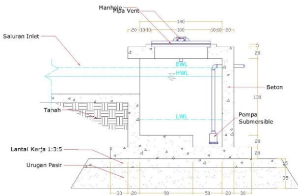
Gambar 3. Potongan Bak Ekualisasi Tanpa Skala
