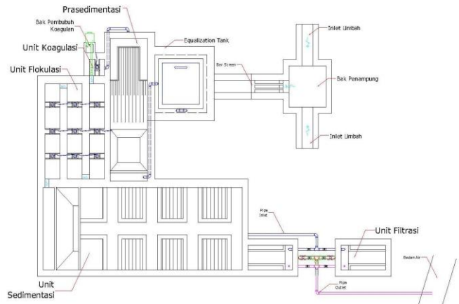
Gambar 1. Layout IPAL Rencana Tanpa Skala
