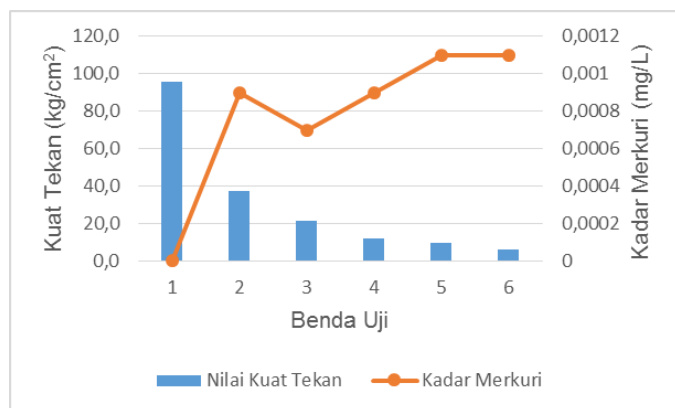
Gambar 4. Grafik Hubungan Kuat Tekan dan Konsentrasi Merkuri
