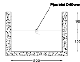
Gambar 13. Potongan Kolam Penampung
