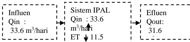
Gambar 6. Kestimbangan massa air
