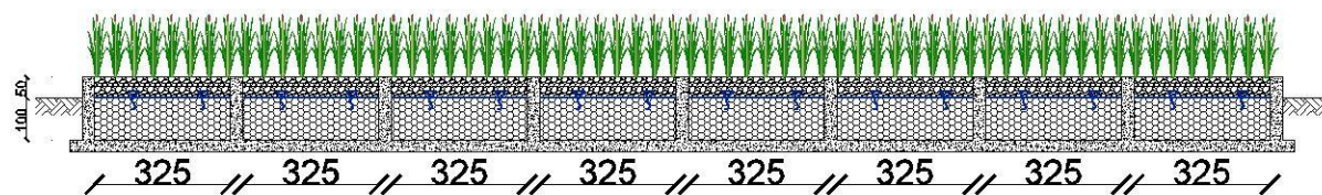
Gambar 8. Potongan B-B unit SSFCW
