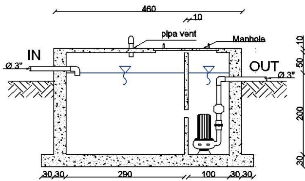
Gambar 6. Potongan A-A bak ekulisasi
