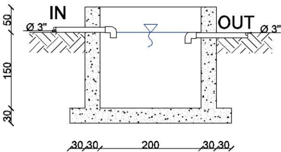
Gambar 10. Potongan melintang kolam indikator
