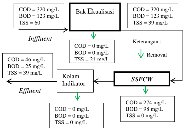
Gambar 1. Mass balance polutan dalam sistem IPAL
