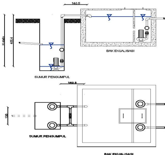
Gambar 3. Skema pemompaan dari bak ekualisasi
