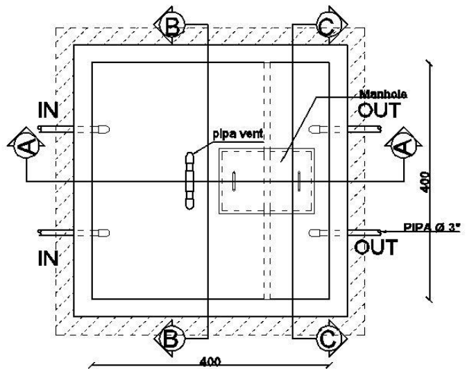
Gambar 5. Denah bak ekualisasi
