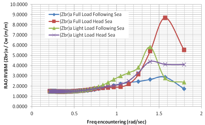
Gambar 11. Grafik RAO gerak vertikal haluan relatif 22 knot
