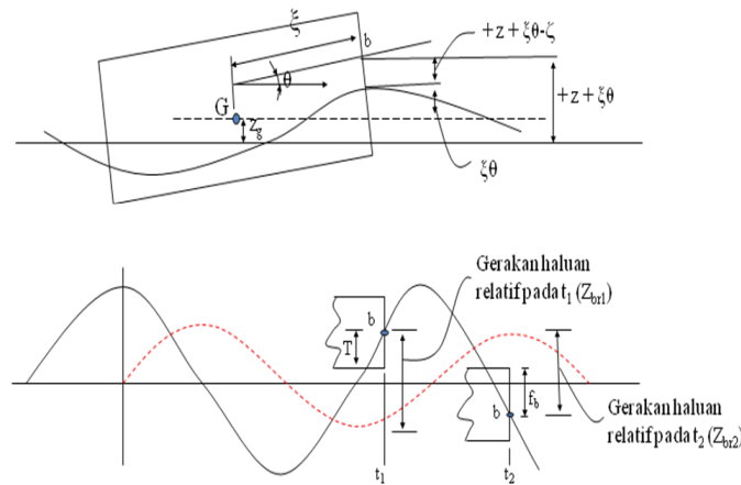
Gambar 6. Definisi gerakan haluan relatif (terhadap gelombang) [8].
