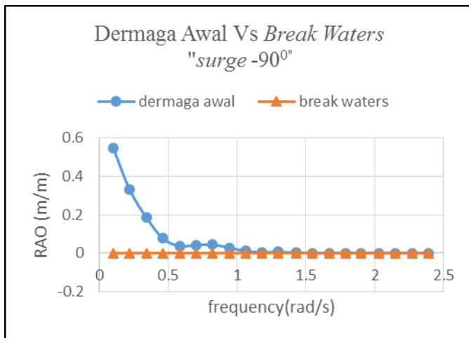
Gambar 9. Perbandingan surging RAO dermaga awal dengan dermaga sebagai break waters
