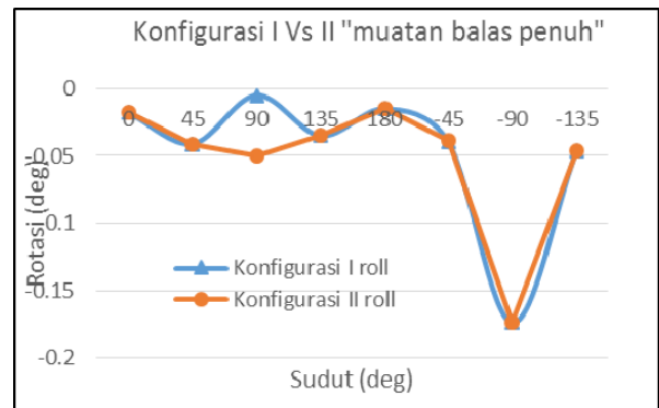
Gambar 7. Grafik perbandingan rolling Konfigurasi I dan II saat muatan balas penuh
