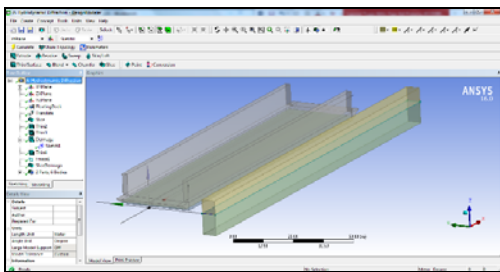
Gambar 3. Pemodelan dok apung dan dermaga pada ansys aqwa
