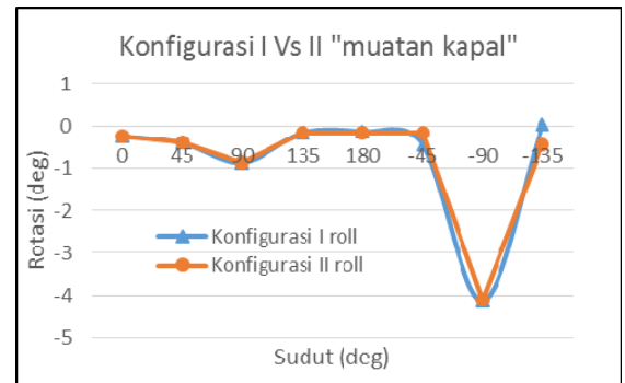
Gambar 6. Grafik perbandingan rolling konfigurasi I dan II saat kondisi muatan kapal
