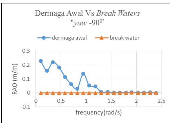
Gambar 11. Perbandingan yawing RAO dermaga awal dengan dermaga sebagai break waters
