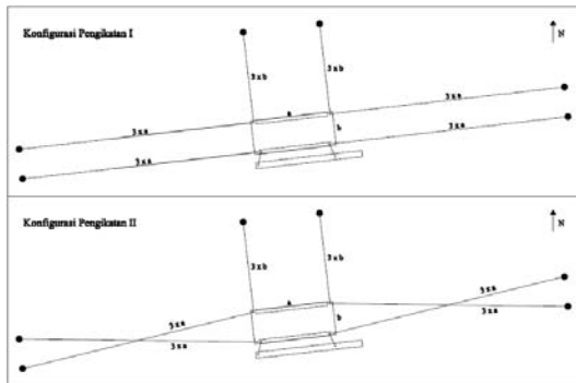
Gambar 4. Variasi Konfigurasi sistem penambatan pada dok apung
