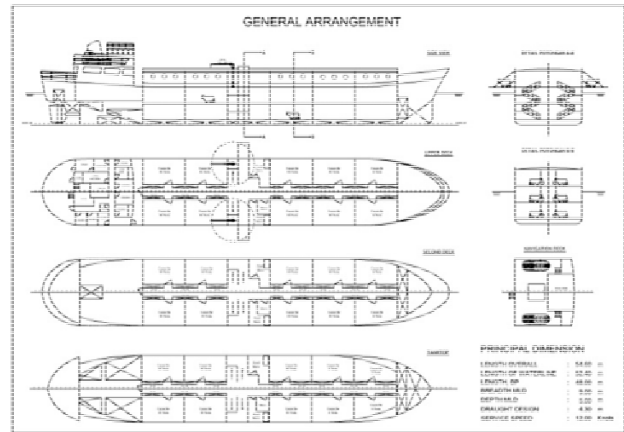
Gambar 6. Rencana Umum Kapal Pengangkut Ternak
