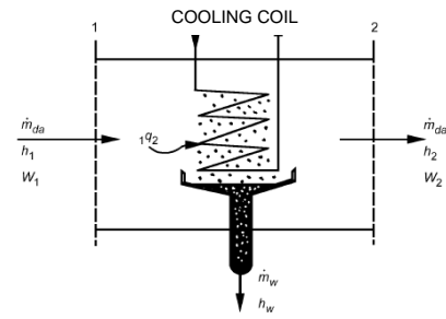
Gambar 3. Skema proses pendinginan
