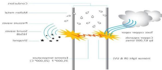
Gambar 1. Efek arc flash .
