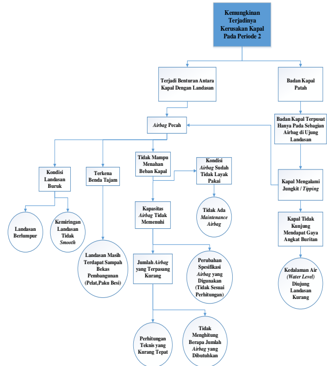
Gambar 7. Kemungkinan terjadinya kerusakan kapal pada periode 2
