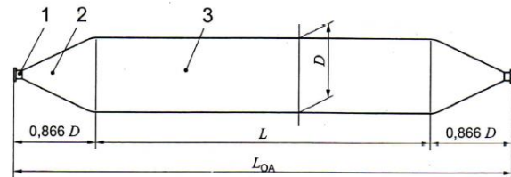
Gambar 3. Struktur airbag [3]
