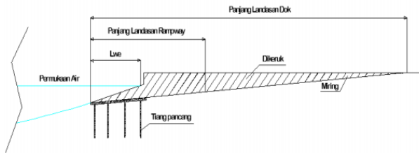
Gambar 1. Skema landasan peluncuran kapal [2]
