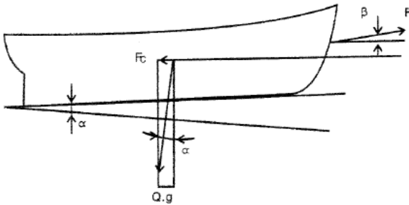
Gambar 4. Gaya yang bekerja pada proses peluncuran kapal dengan airbag [3]
