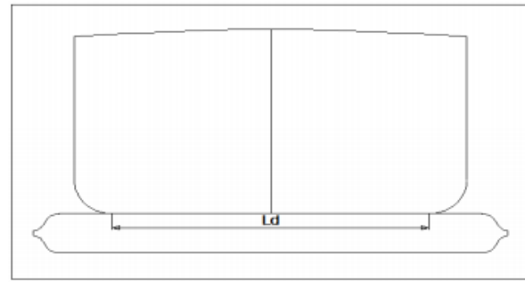
Gambar 2. Panjang kontak antara airbag dan lunas kapal (L D ) [3]
