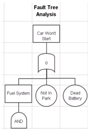
Gambar 5. Contoh penggunaan FTA [5]
