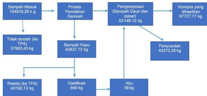
Gambar. 2. Diagram alir Material Balance skenario kedua
