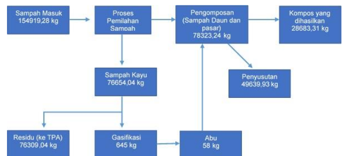
Gambar. 1. Diagram alir Material Balance skenario pertama
