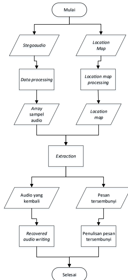
Gambar 2. Diagram alir yang menunjukkan alir proses extraction pada perangkat lunak.
