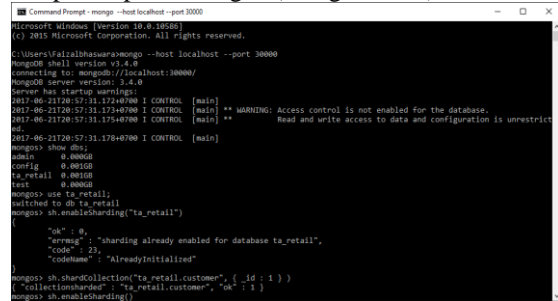
Gambar 18. Penampang Mongos dari Sharding
