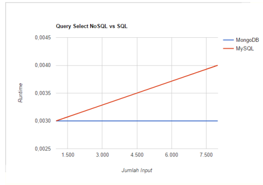
Gambar 10. Grafik Perbandingan Runtime Select
