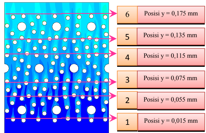
Gambar 10. Posisi pengambilan data input untuk psychometric chart
