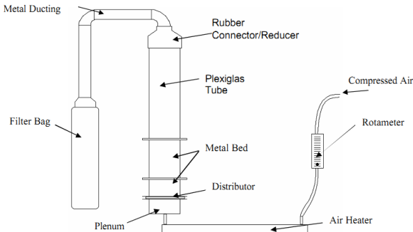
Gambar 2. Skema Alat Ekperimental Penelitian
