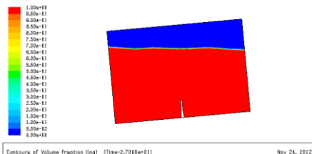
Gambar 15. gerakan fluida pada volume 75% tangki dengan baffle
