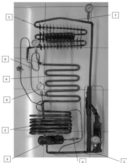
Gambar 2 Hasil Modifikasi Evaporator dan Generator [2]
