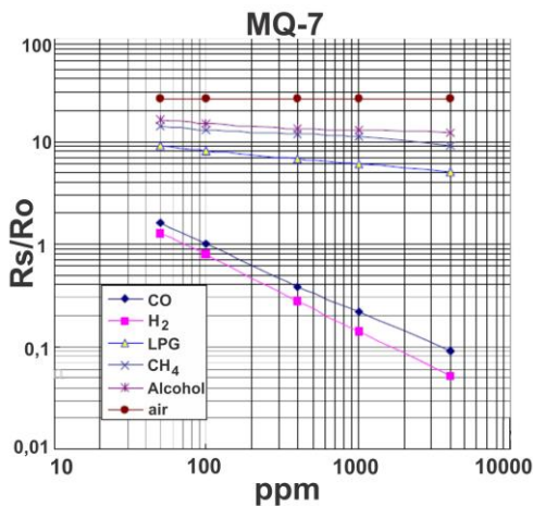
Gambar 1. Grafik Sensitifitas Sensor MQ-7 [1].
