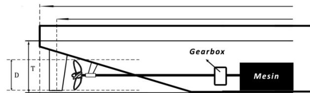
Gambar 4. Sketsa penempatan propeler pada barge
