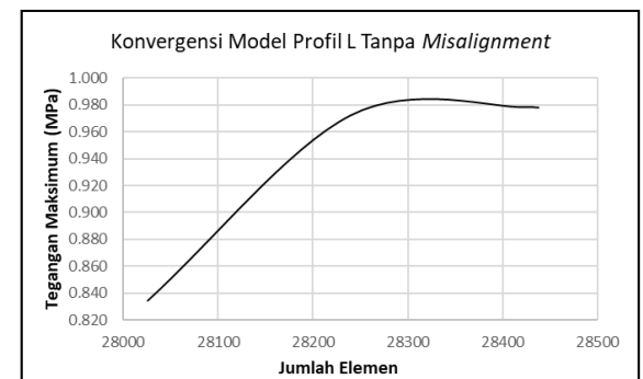
Gambar 4. Konvergensi model profil L tanpa misalignment
