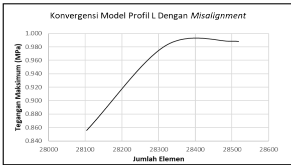
Gambar 5. Konvergensi model profil L dengan misalignment .
