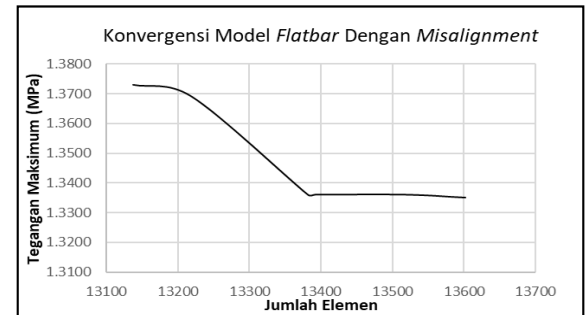
Gambar 3. Konvergensi model flatbar dengan misalignment .
