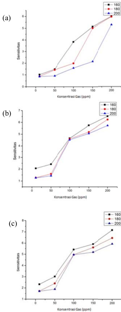
Gambar 7. Menunjukkan pengaruh konsentrasi gas LPG terhadap sensitivitas sensor untuk temperatur operasi a) 30°C, b) 50°C dan c) 100°C
