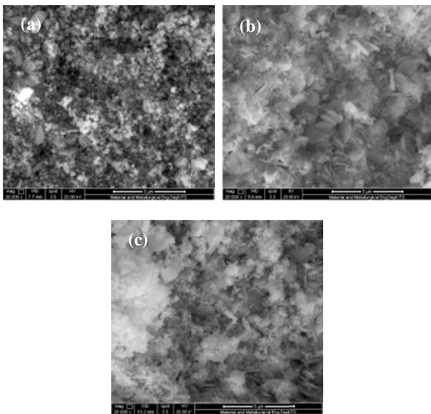
Gambar. 2. Hasil Uji SEM untuk pellet WO 3 setelah terpapar gas LPG pada perbesaran 20000x untuk temperatur post hydrothermal a) 160 °C, b) 180 °C, dan c) 200 °C.
