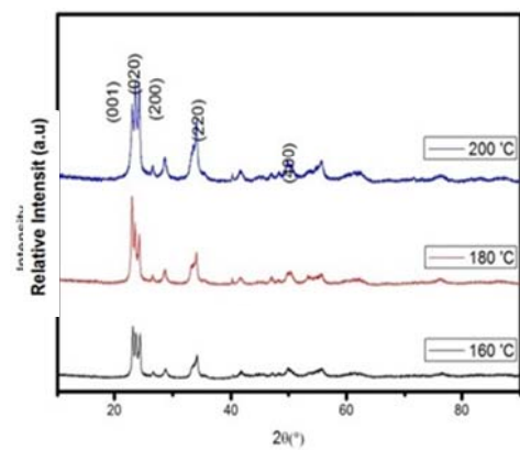
Gambar 4. Hasil pengujian XRD pellet WO 3 setelah terpapar gas LPG.
