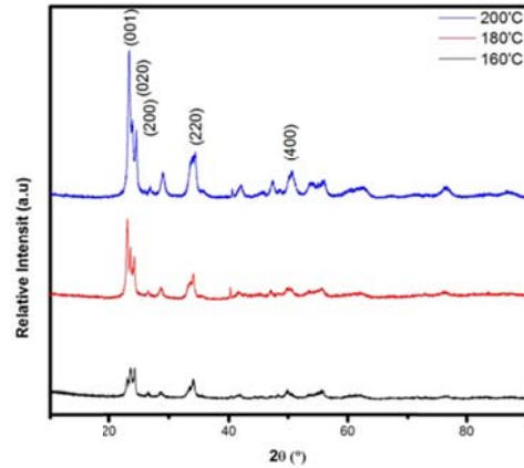
Gambar. 3. Hasil pengujian XRD pellet WO 3 sebelum terpapar gas LPG.
