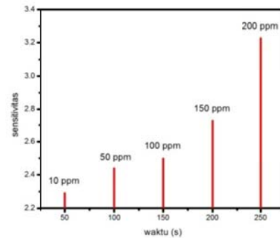
Gambar 8. Menunjukkan nilai respon dinamis untuk material WO 3 dengan temperature post hydrothermal 160°C dan temperature operasi 100°C.
