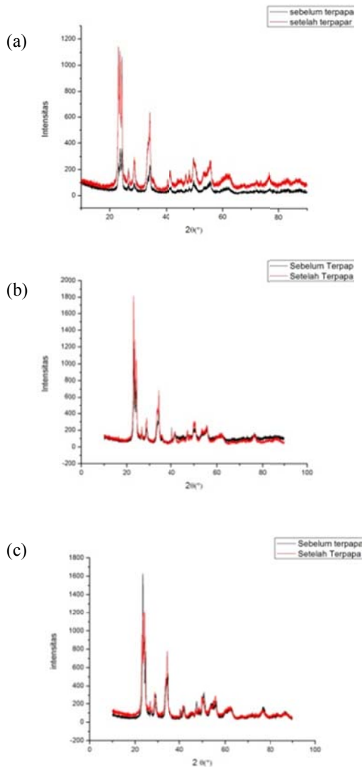
Gambar 5. Hasil perbandingan grafik XRD sensor WO 3 sebelum dan sesudah terpapar gas LPG untuk variasi temperature post hydrothermal a)160°C, b) 180°C, dan c)200°C.
