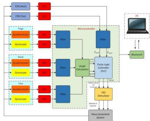
Gambar 1. Diagram blok keseluruhan sistem
