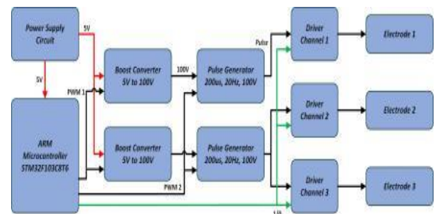
Gambar 2. Diagram blok keseluruhan sistem FES
