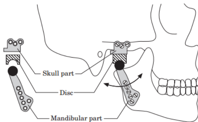
Gambar. 1. Desain dasar dari Groningen prosthesis TMJ, terdiri dari bagian fossa , bagian mandibular , dan disc yang bersinggungan [1].
