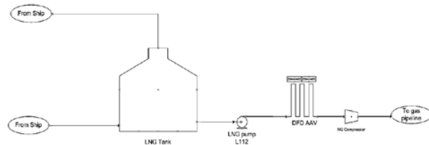
Gambar 7. Process Flow Diagram Proses Regasifikasi dengan Direct Forced Draft Ambient Air Vaporizer
