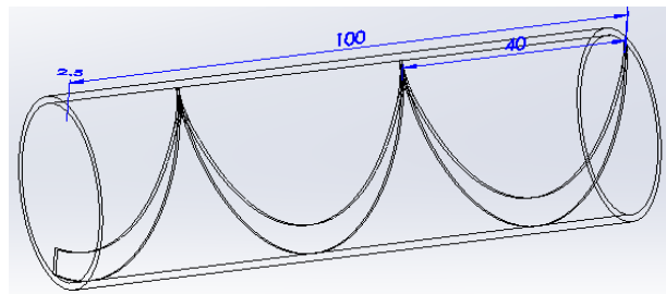
Gambar 2 Intake Manifold dengan Ulir 1
