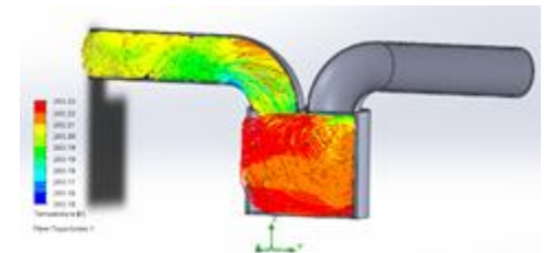
Gambar 7 Analisa Aliran pada Intake Manifold dengan Penambahan Ulir Kedua
