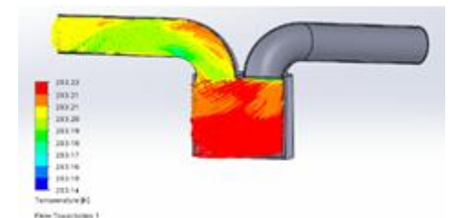
Gambar 8 Analisa Aliran pada Intake Manifold dengan Penambahan Ulir Ketiga
