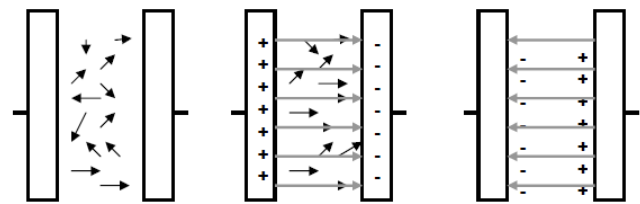
Sebelum adanya muatan pada kedua pelat, bahan dielektrik memiliki dipole acak sehingga bersifat isolator
