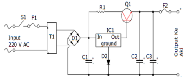
Gambar 4 Desain modifikasi rangkaian baterai charger
