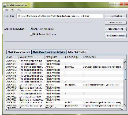
Gambar 3. Antarmuka Kakas Bantu Saat Melakukan Pengujian Fungsional
