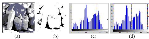
Gambar 10. Citra Peppers dengan 5 Ambang (a) Hasil Metode Median-based Otsu dengan Nilai Ambang 48, 86, 121, 152, dan 172 (b) Hasil Metode Median-based MET dengan Nilai Ambang 2, 46, 132, 246 dan 248 (c) Histogram Hasil Metode Median-based Otsu (d) Histogram Hasil Metode Metode Median-based MET
